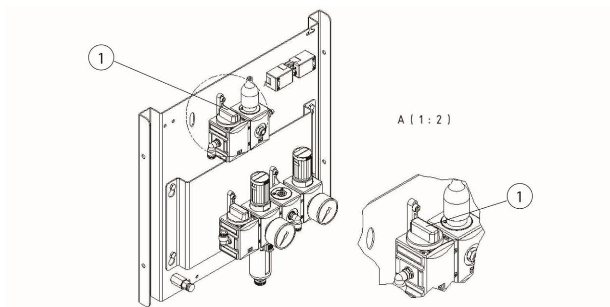
Fig. 37 : soupape pneumatique bac collecteur de poussières
